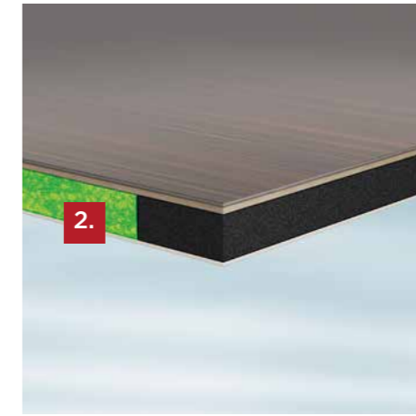
2. Spezieller Isolierkern aus XPS-Schaum für eine perfekte Dämmung
