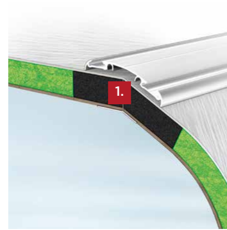
1. Extraharter PU-Kern für eine hohe Schlagfestigkeit
